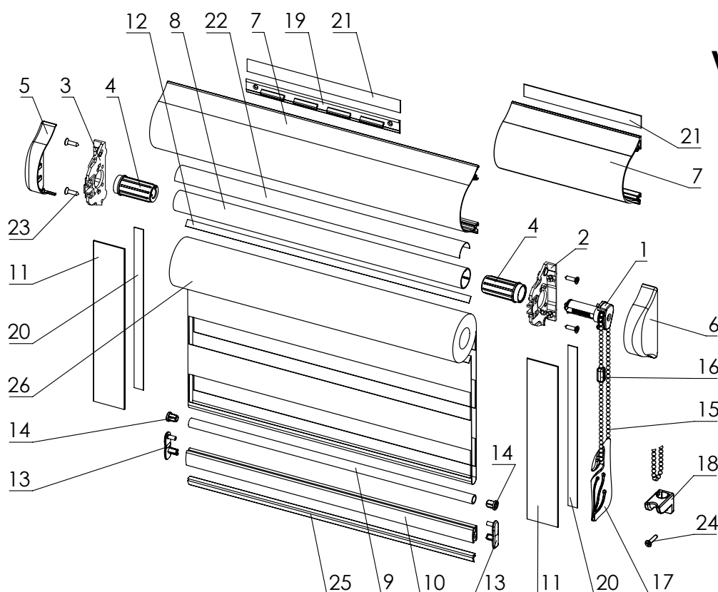
Schemat i wykaz elementów rolety Vegas Classic XL (wykonanie Dzień i Noc, rura 18 mm, mechanizm Vegas)
