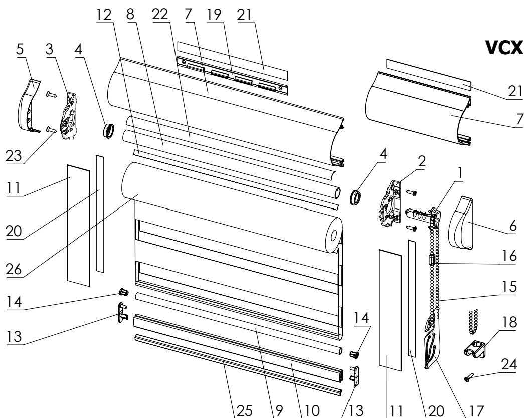
Schemat i wykaz elementów rolety Vegas Classic XL (wykonanie Dzień i Noc, rura 13,5 mm, mechanizm Klaudia)
