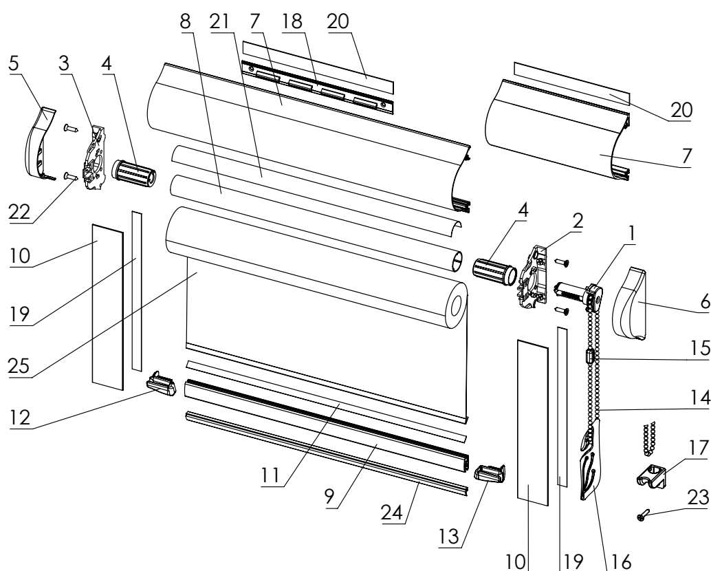
Schemat i wykaz elementów rolety Vegas Classic XL (wykonanie standard, rura 18 mm, mechanizm Vegas)
