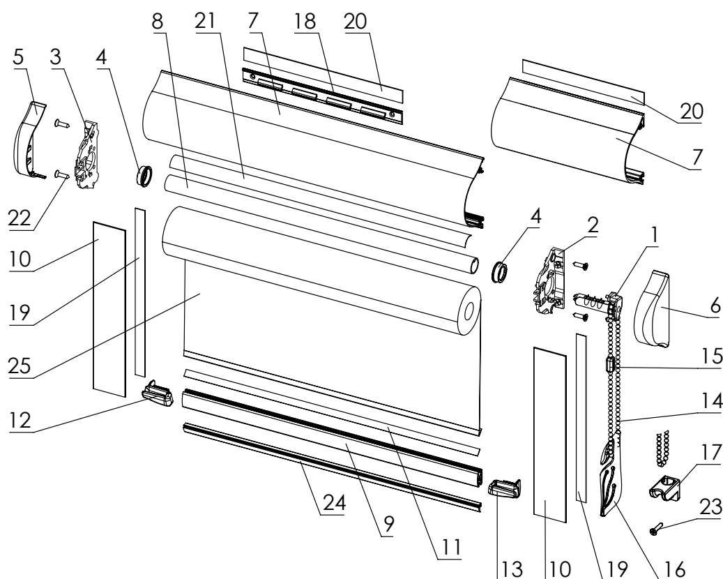
Schemat i wykaz elementów rolety Vegas Classic XL (wykonanie standard, rura 13,5 mm, mechanizm Klaudia)
